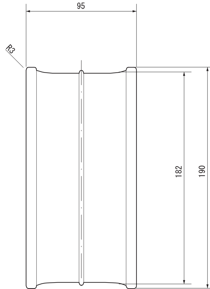
【側面図】
