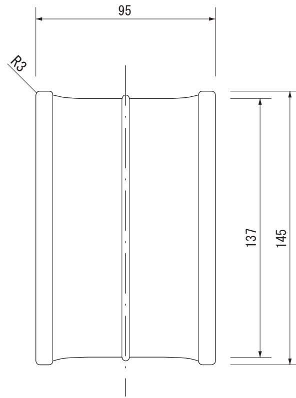
【側面図】
