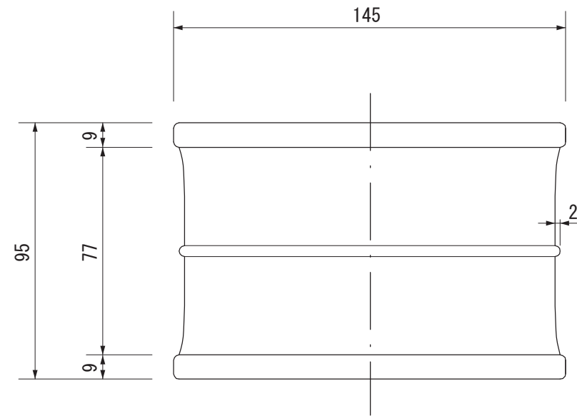
【上面図】
