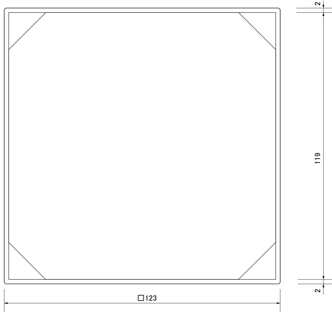
【上面図】
