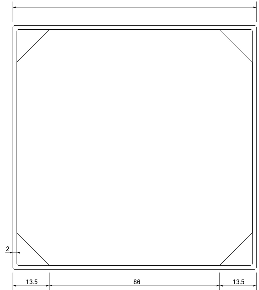
【底面図】
