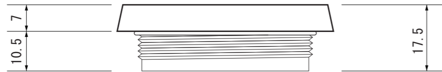
【側面図】
