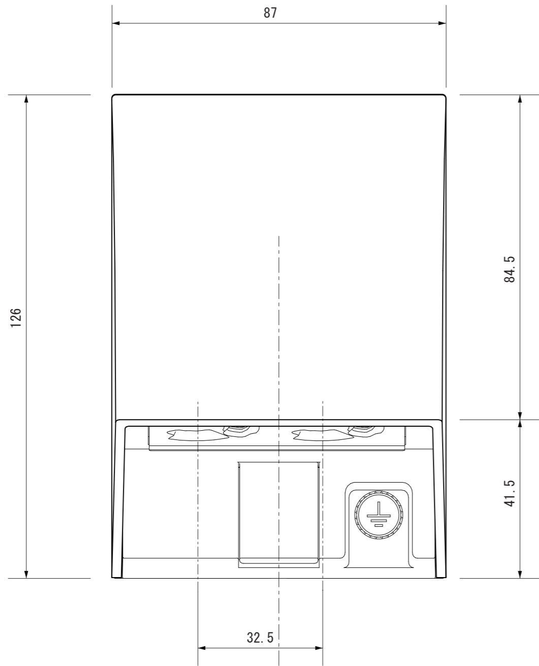
【正面図】
