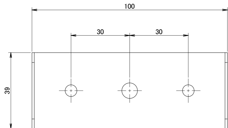
1 【本体】
