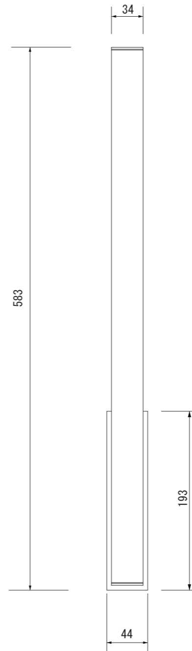
【正面図】
