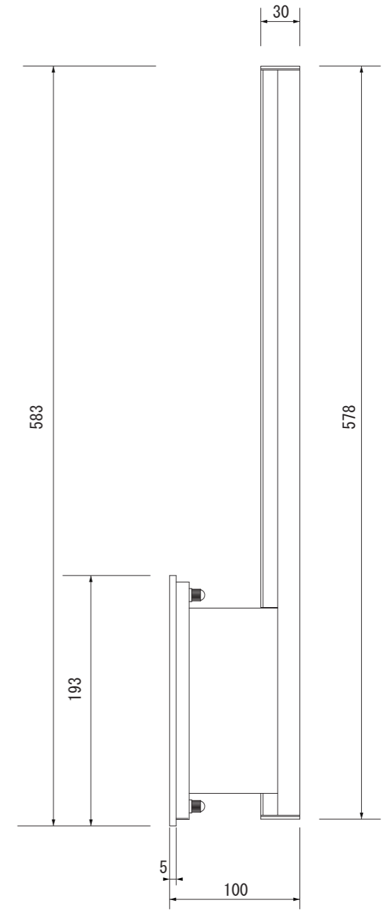
【側面図】
