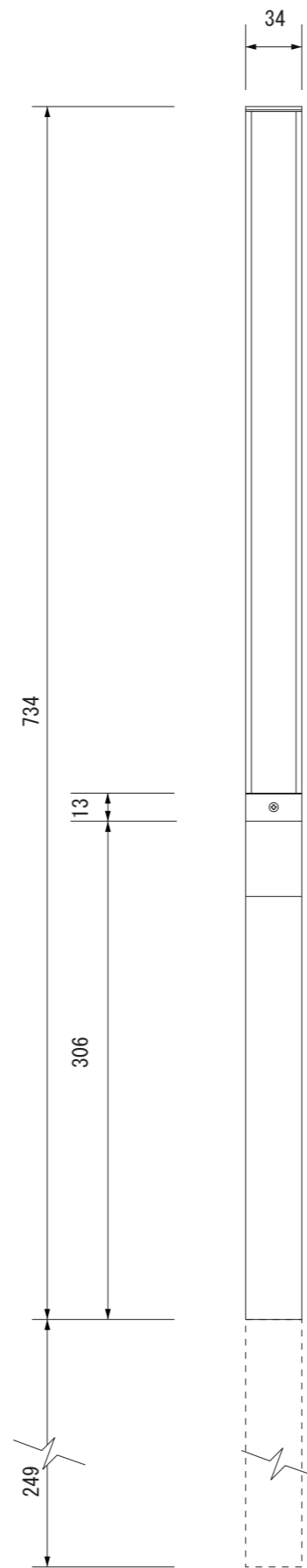
【正面図】
