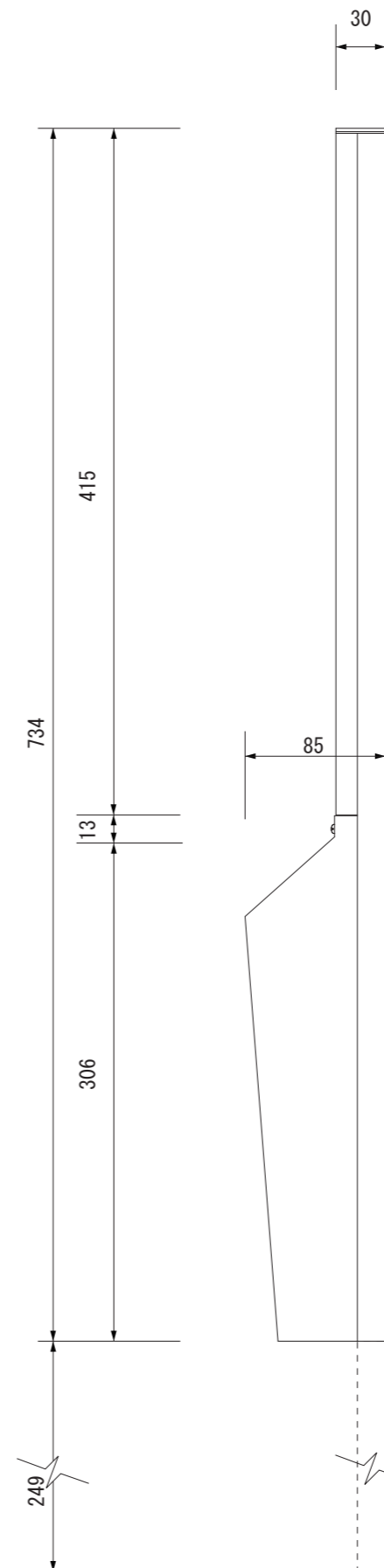
【側面図】
