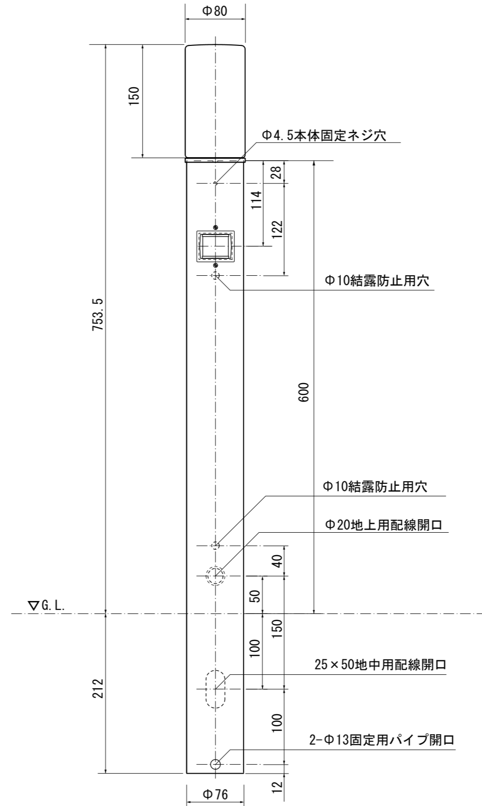
【正面図】
