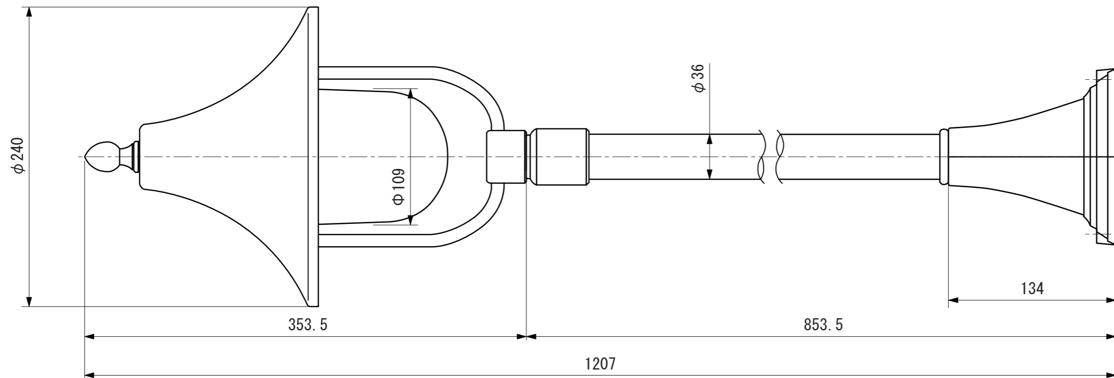
【正面】
