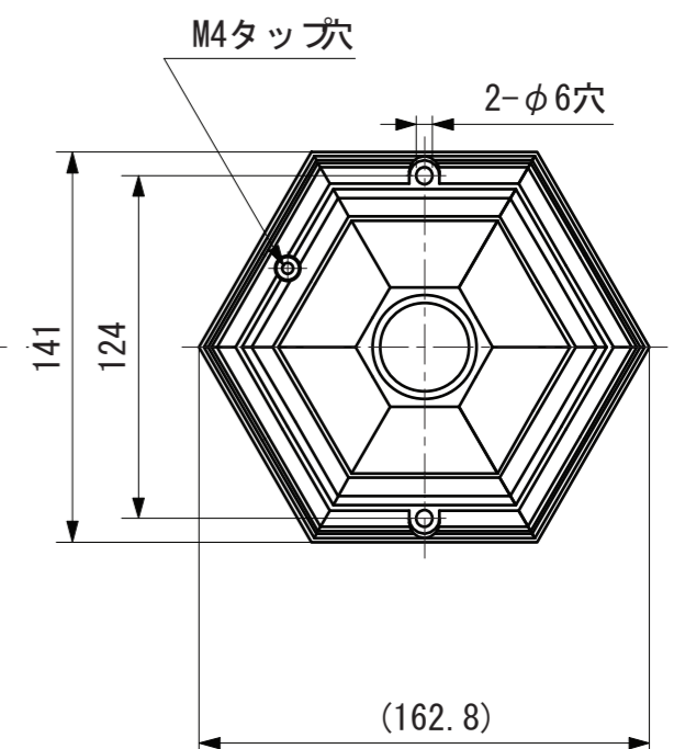
【底面】
