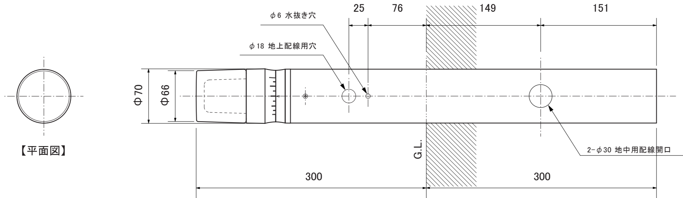
【正面図】
