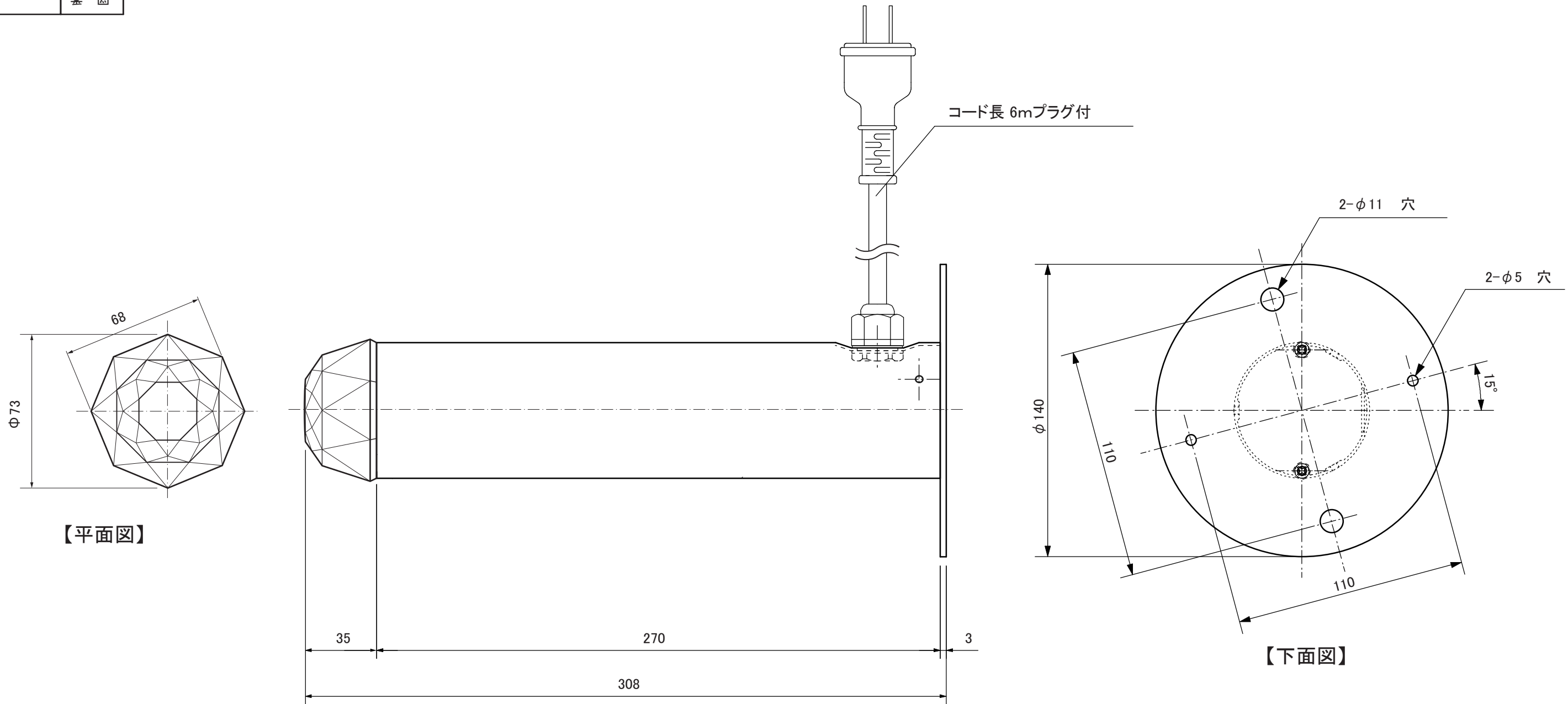
【正面図】
