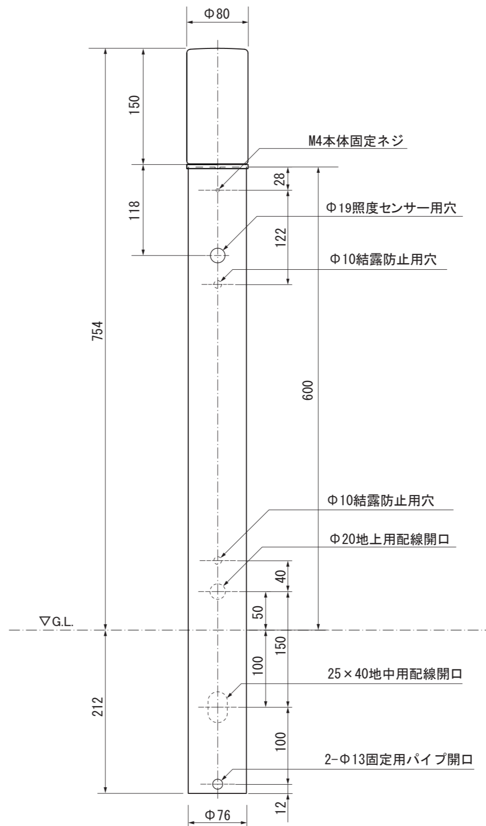
【正面図】
