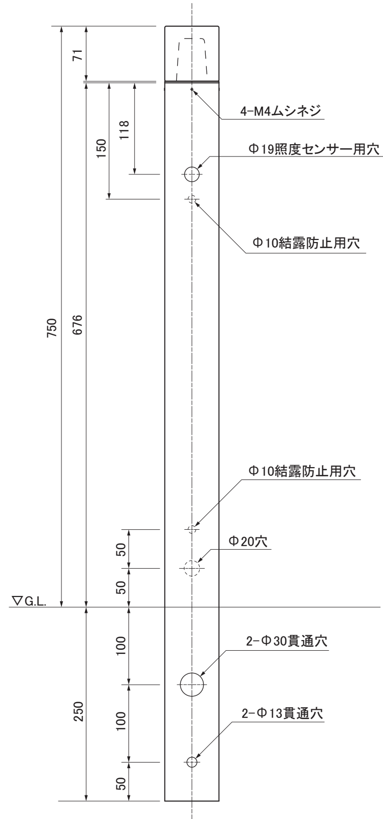
【正面図】
