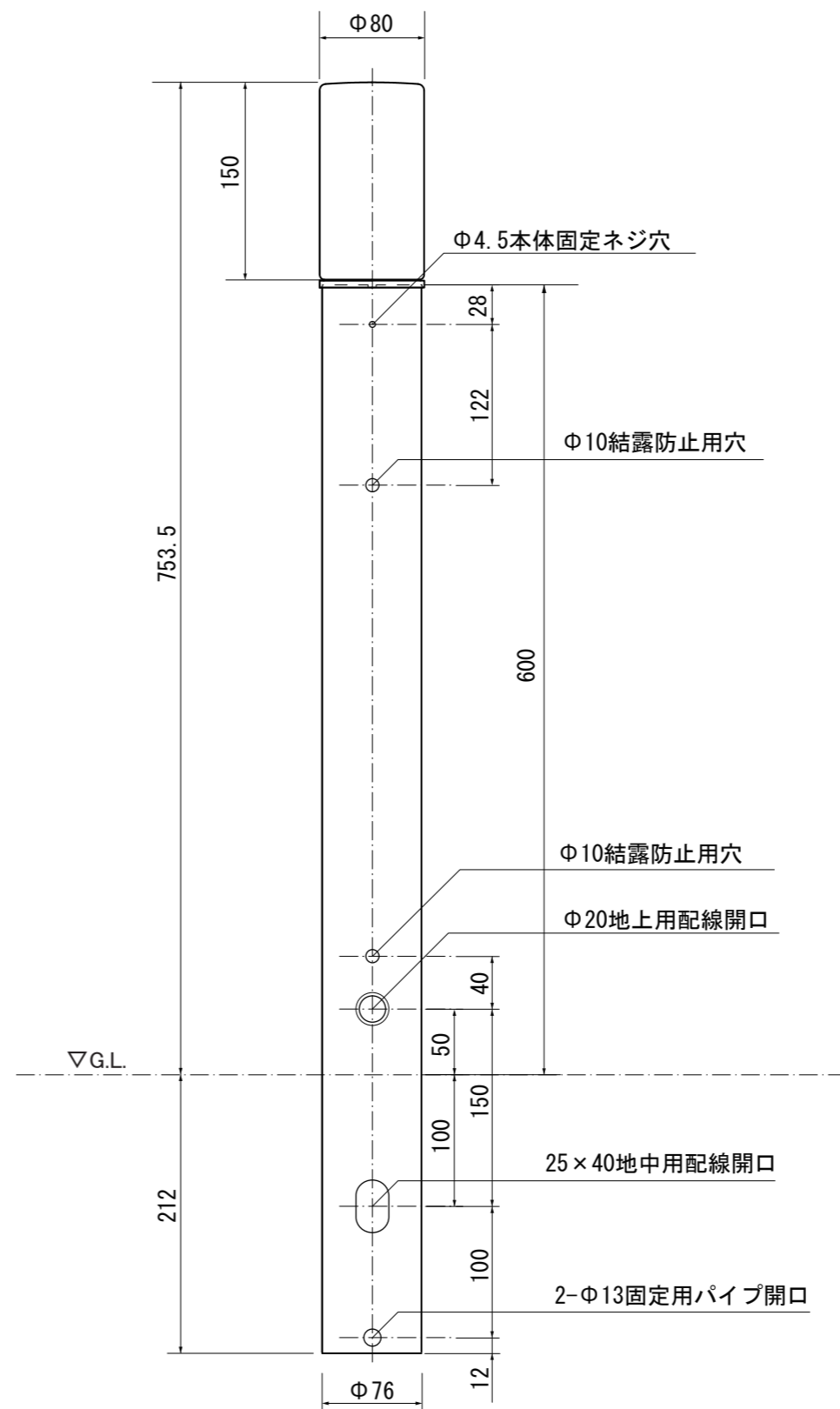
【正面図】
