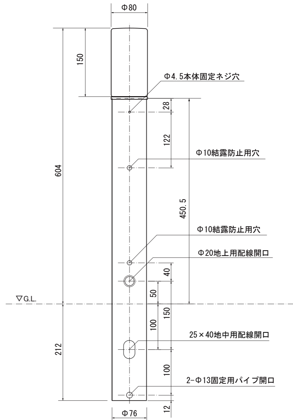
【正面図】
