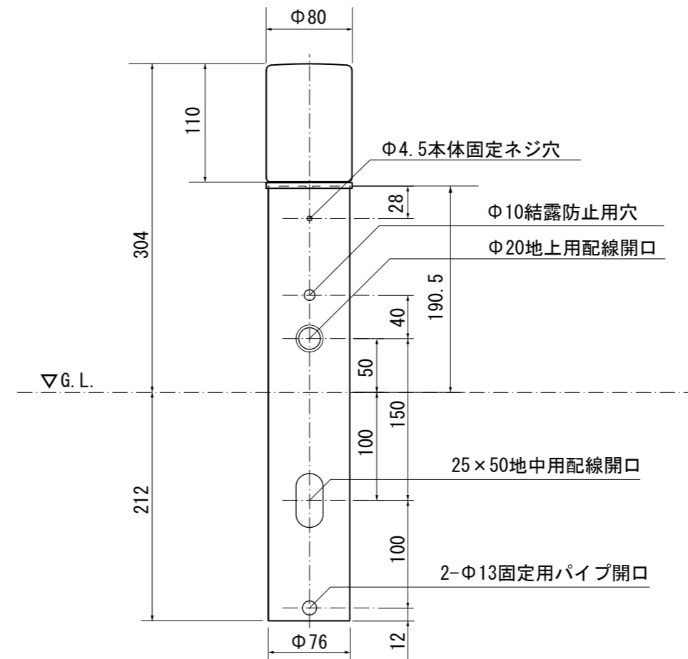
【正面図】
