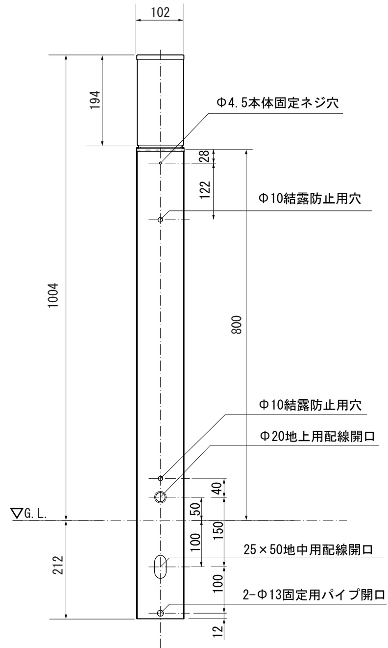
【正面図】
