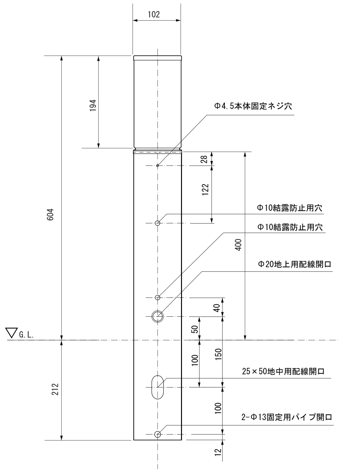
【正面図】
