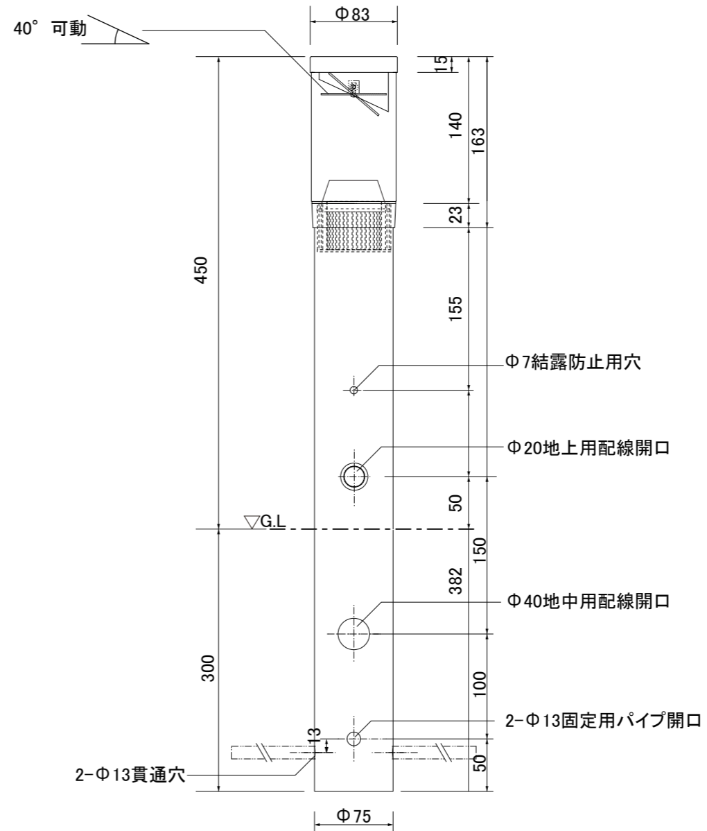
【正面図】
