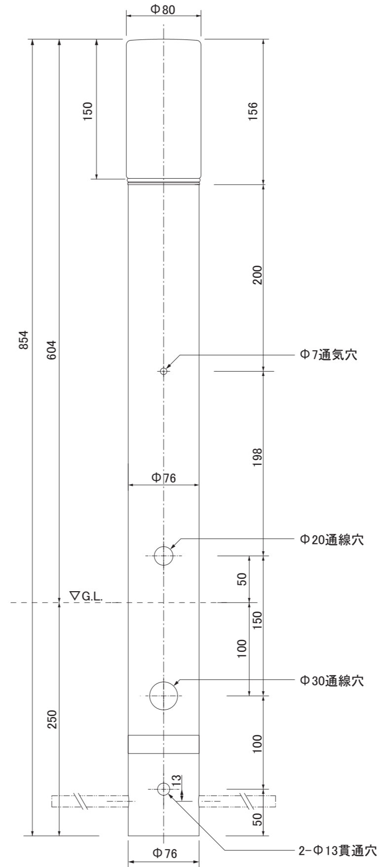
【正面図】
