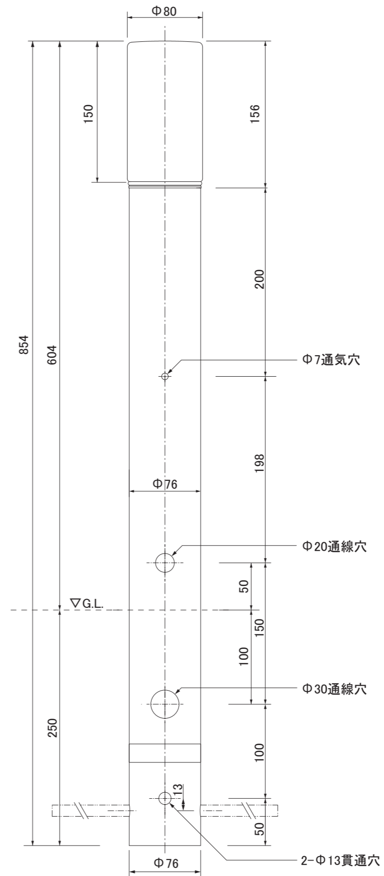
【正面図】
