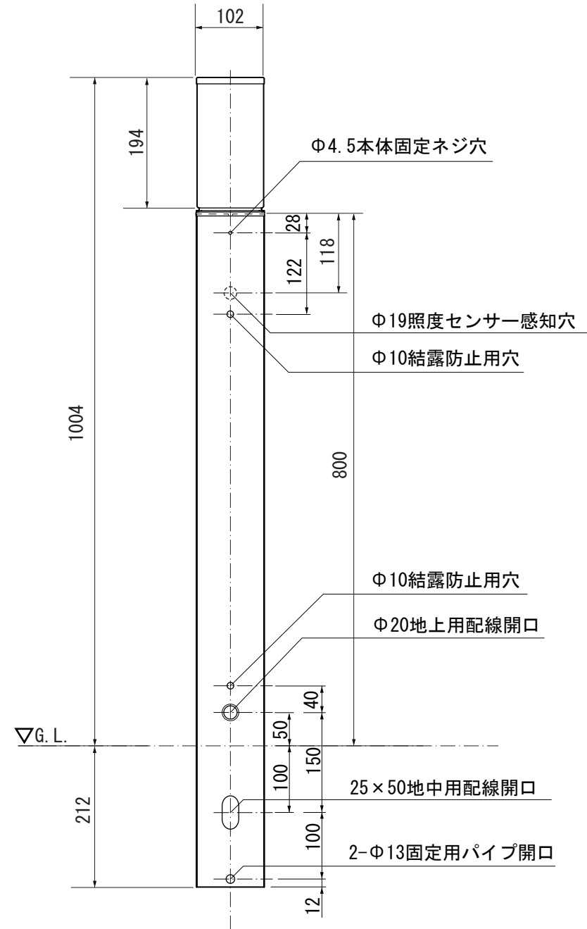
【正面図】
