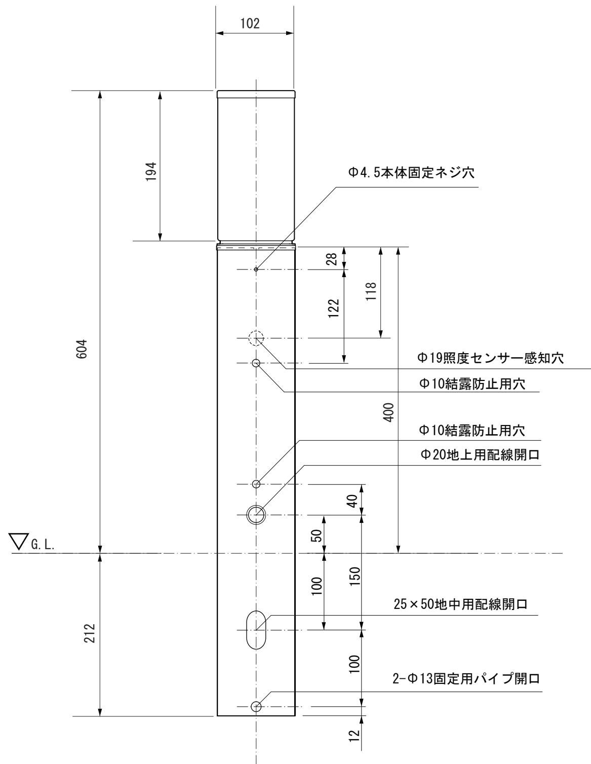
【正面図】
