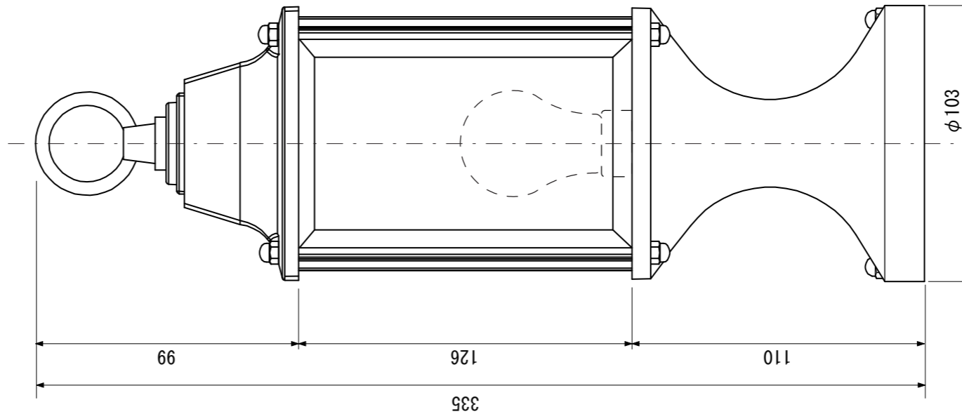
【正面図】
