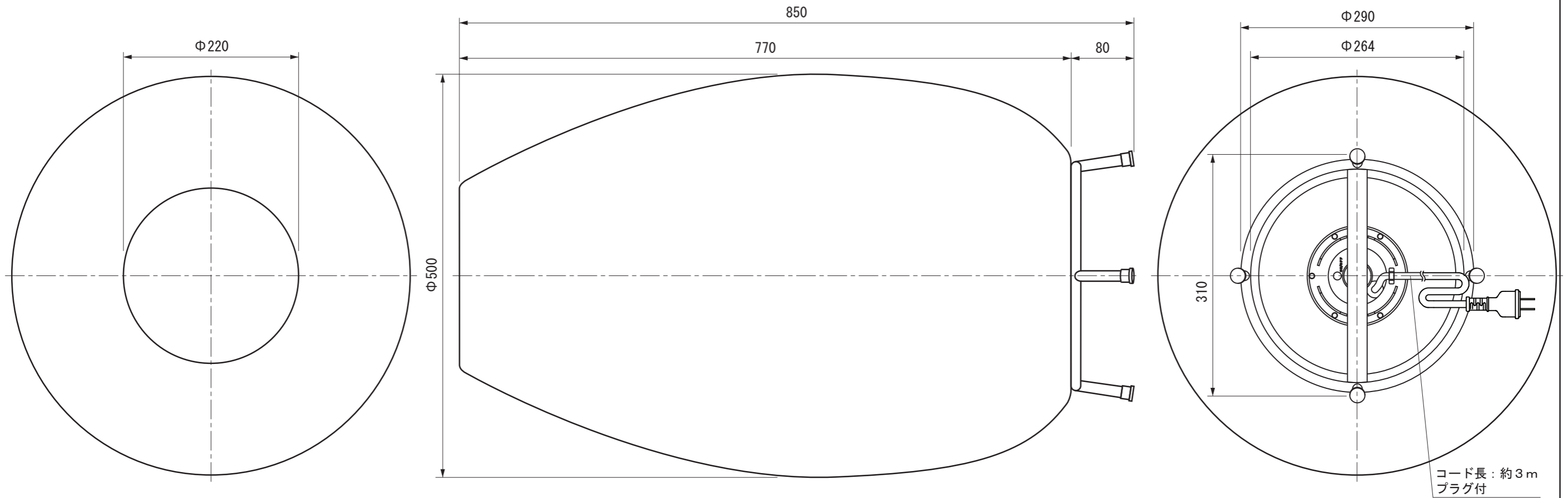
【上面図】
