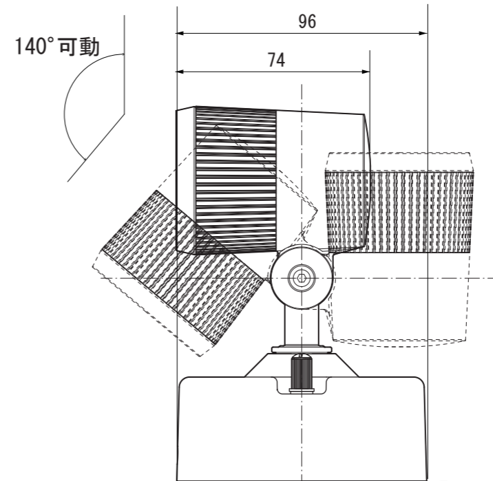
【側面図】
