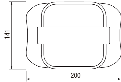
【上面図】
