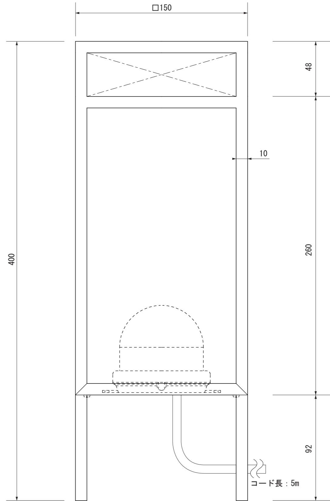
【正面図】
