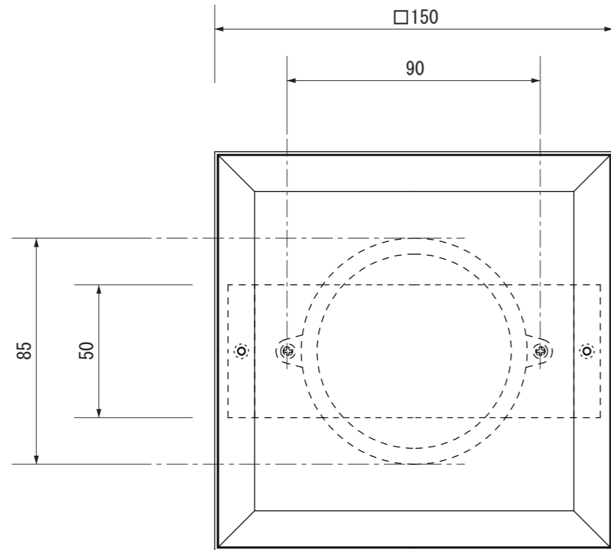
【上面図】
