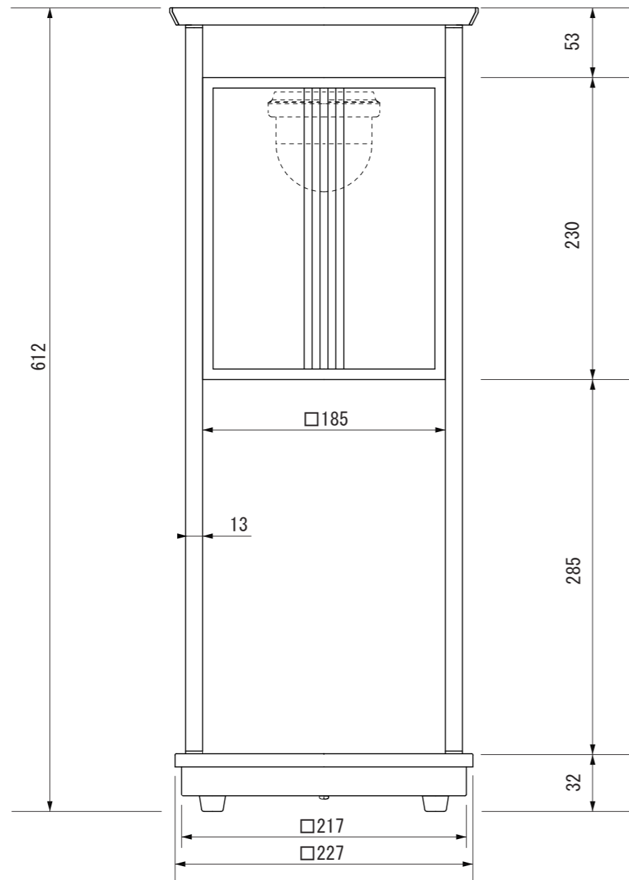
【正面図】
