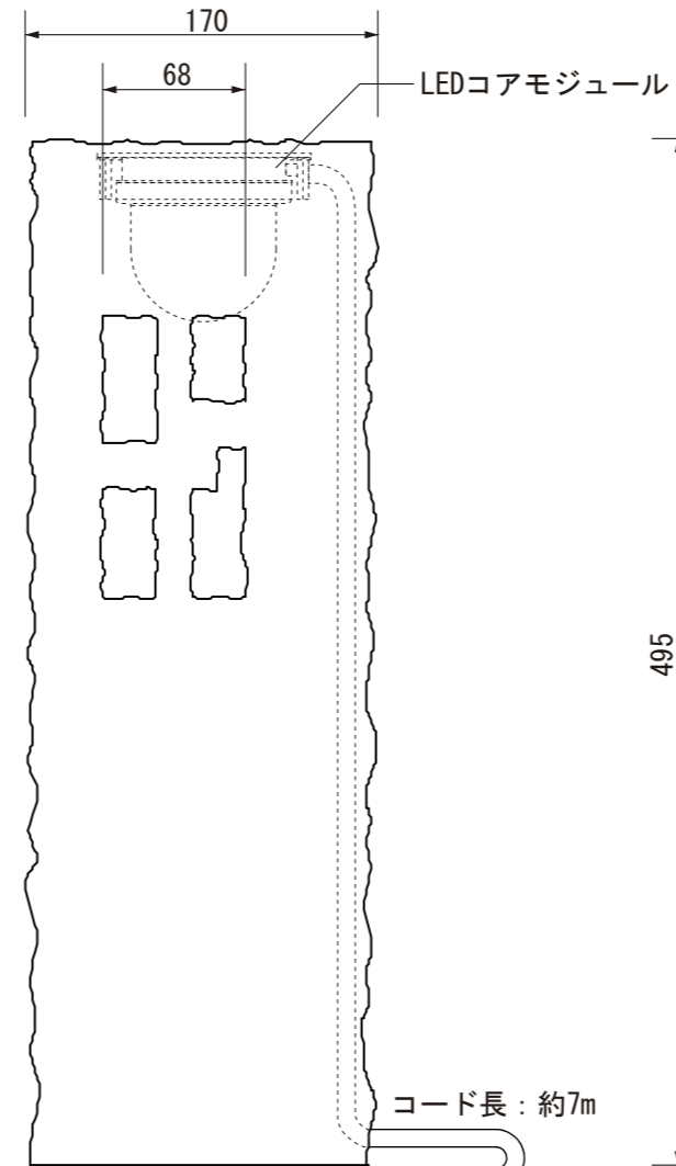
【右側面図】
