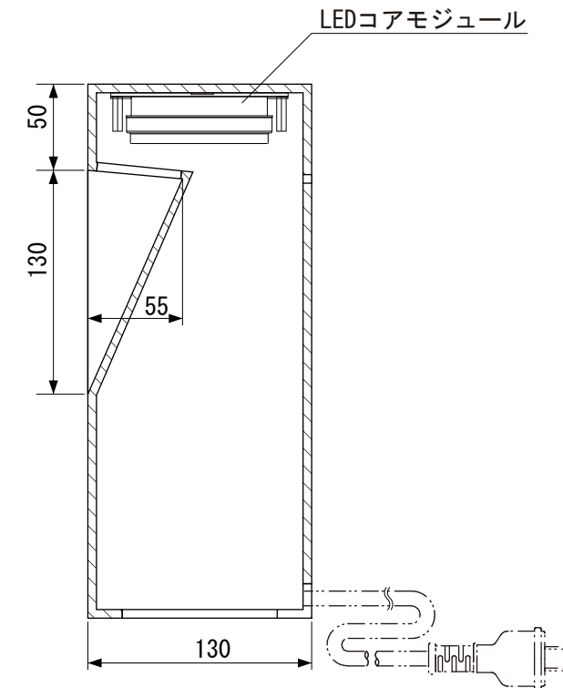
【断面図】
