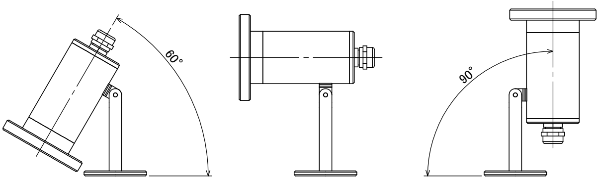
首振り可動範囲(150度)
