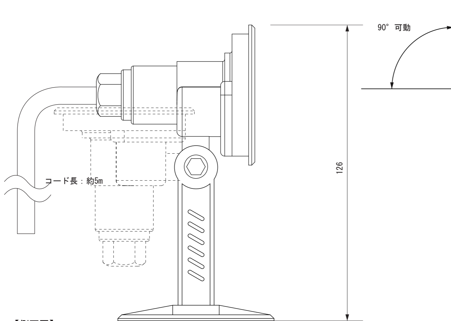
【側面図】
