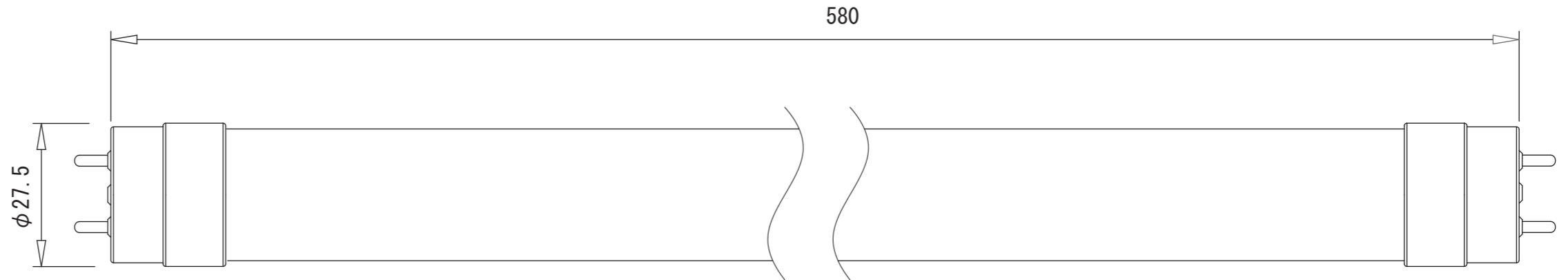
【正面図】
