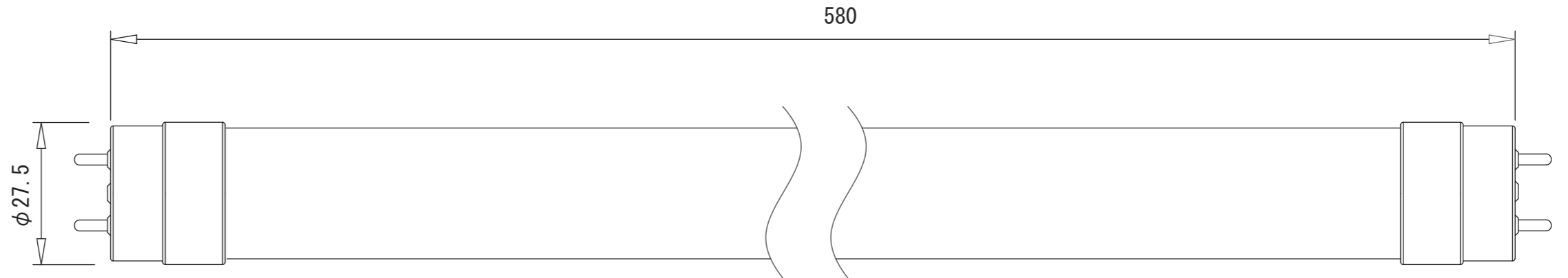
【正面図】
