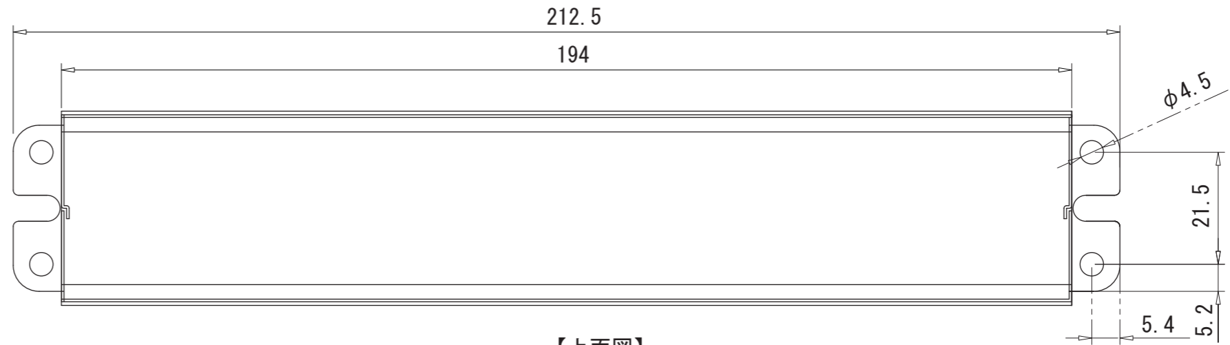
【上面図】
