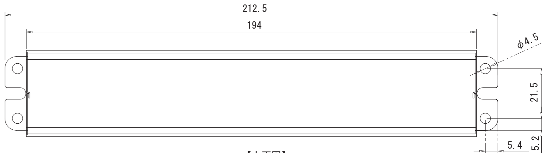
【上面図】
