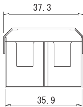
【側面図】
