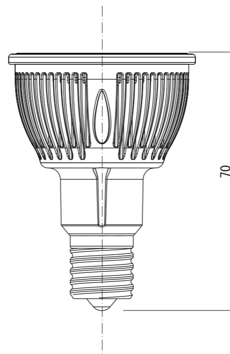
【正面図】
