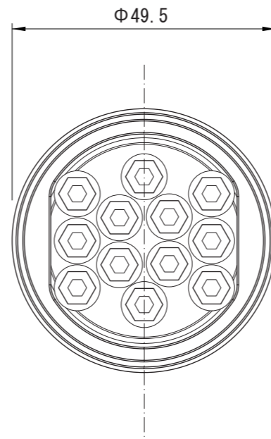
【上面図】
