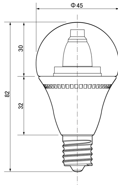
【正面図】
