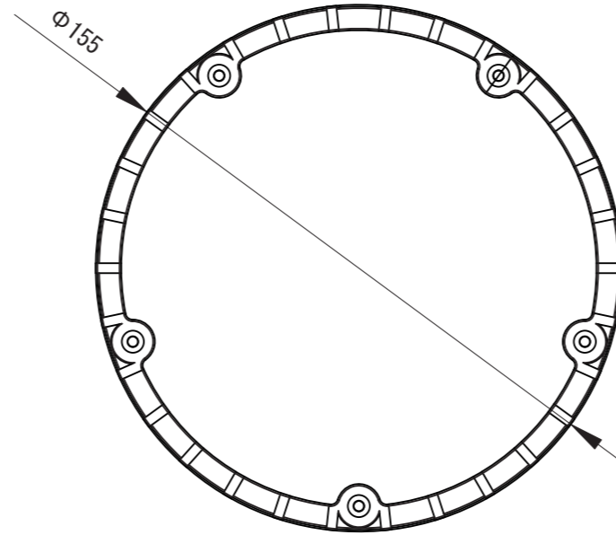
【上面図】
