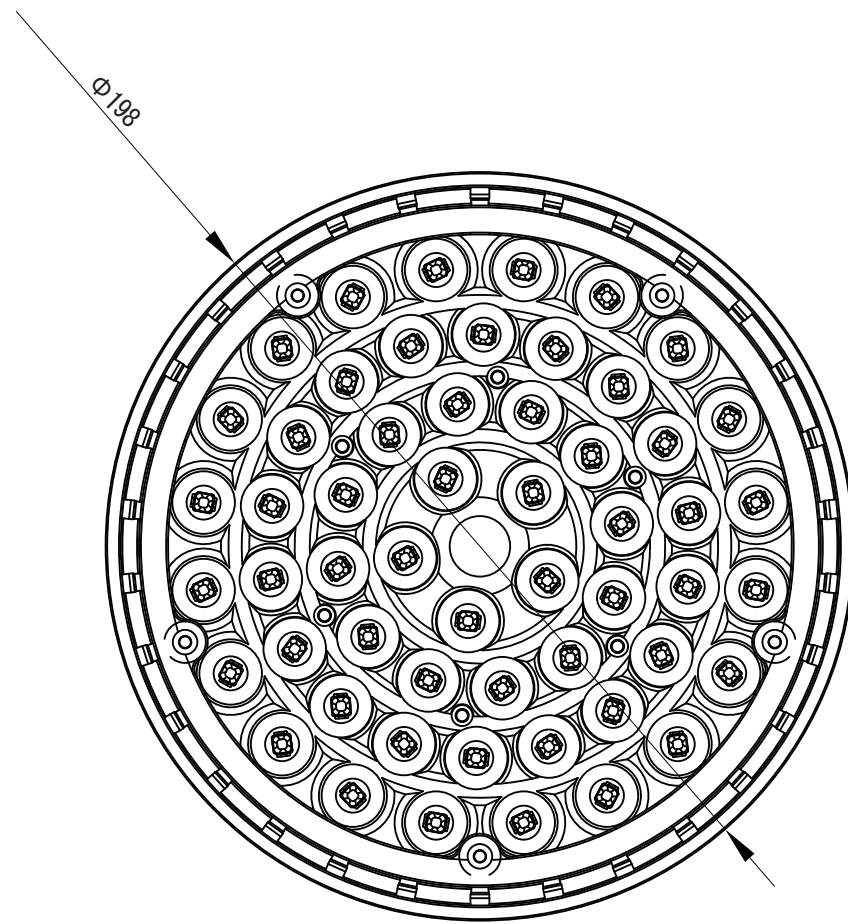
【上面図】
