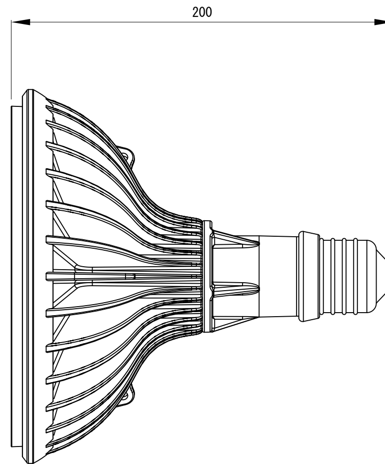
【正面図】
