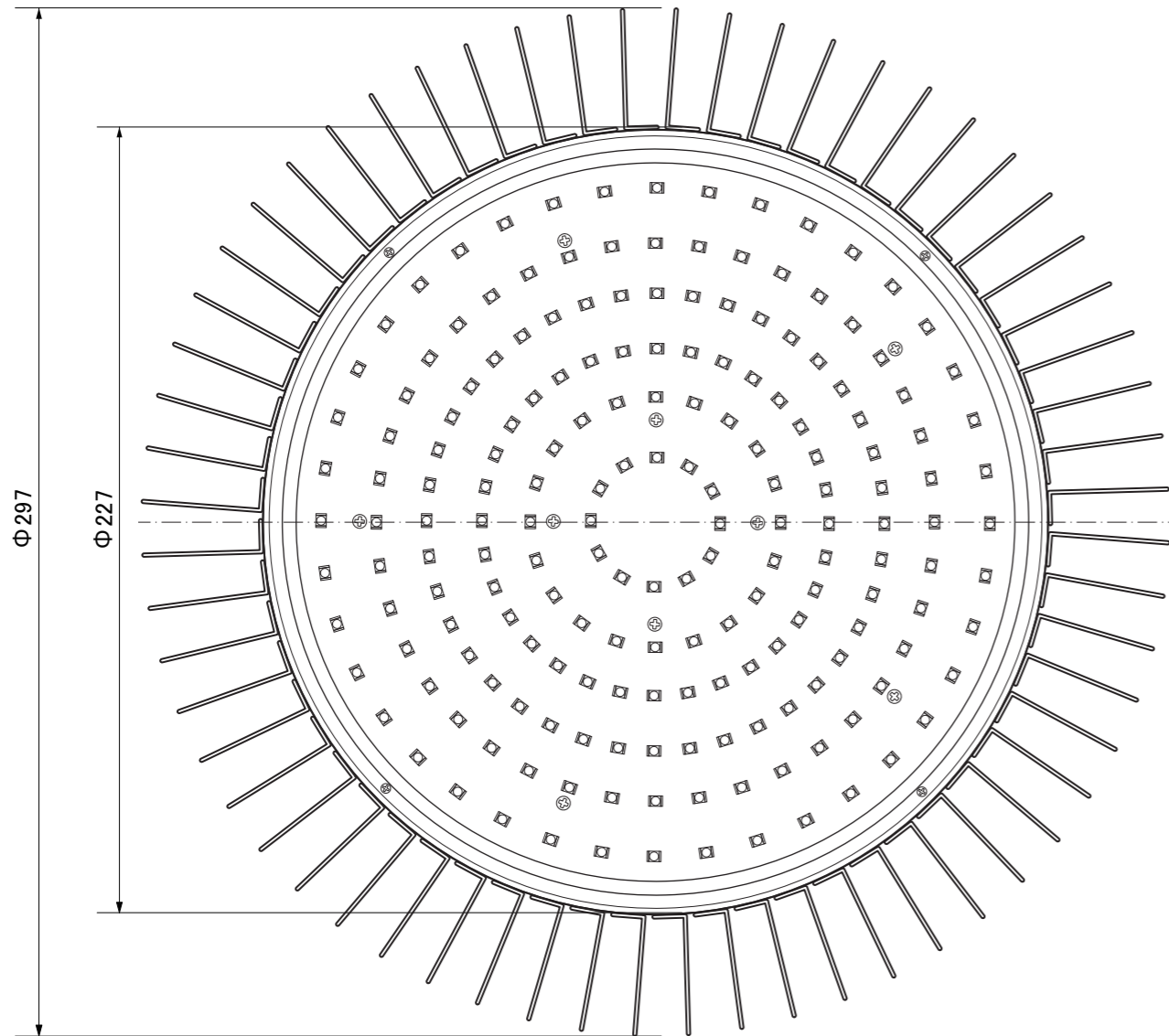
【上面図】
