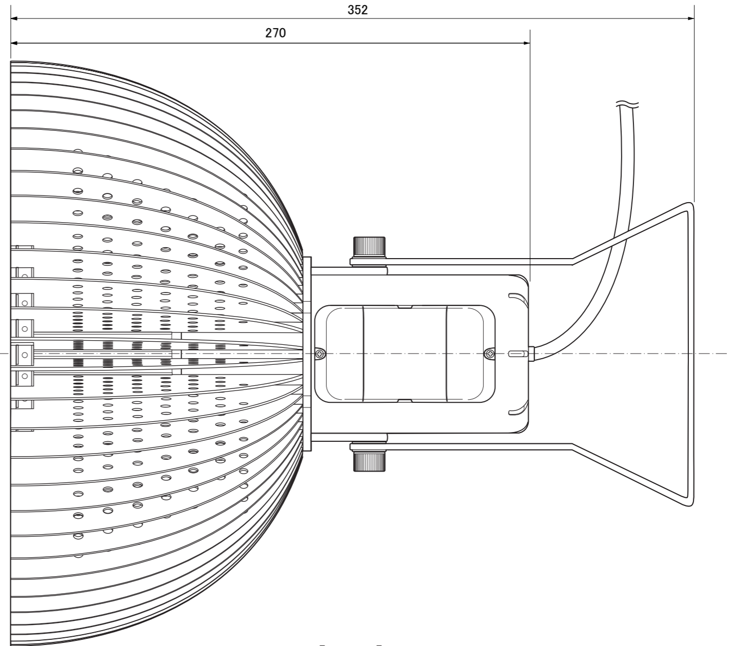
【正面図】
