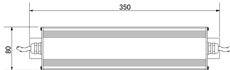
【上面図】
