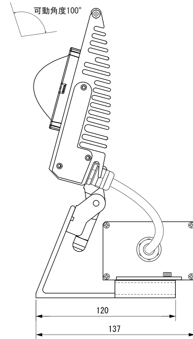
【側面図】
