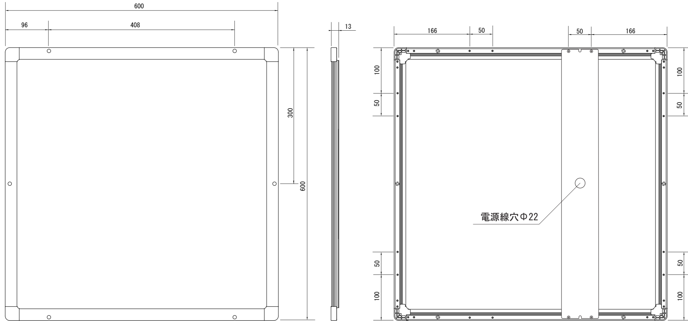
【正面図】
