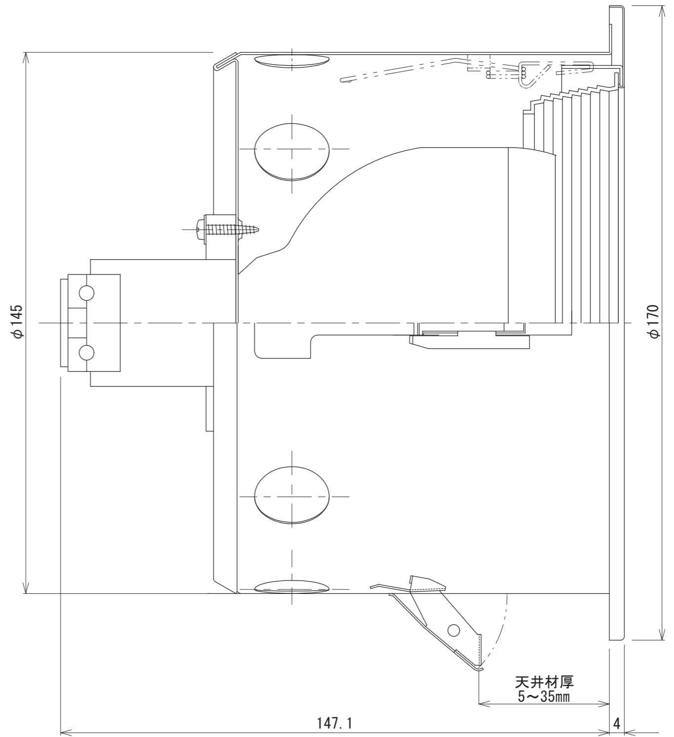
【側面図】
