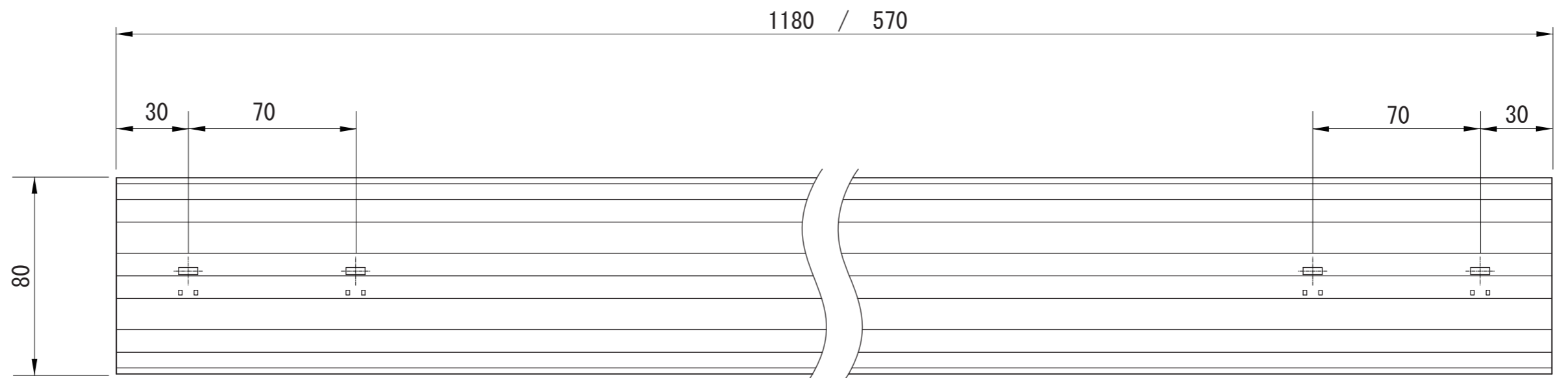
【正面図】
