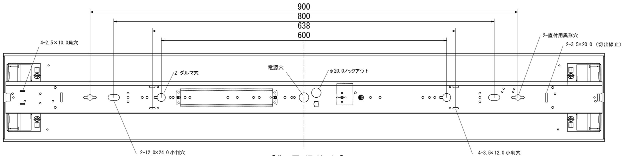
【背面図（取付面）】
