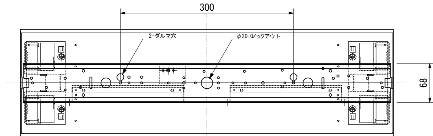
【背面図（取付面）】
